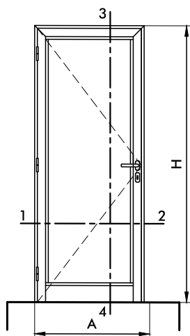
VISTA PUERTA DE ABRIR 1 HOJA ESCALONADA CONTRAVIDRIOS RECTOS
