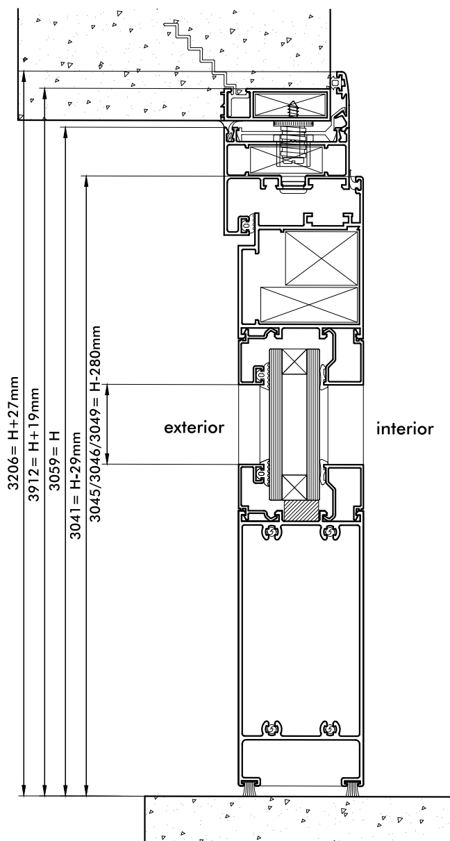
CORTE 3-4
